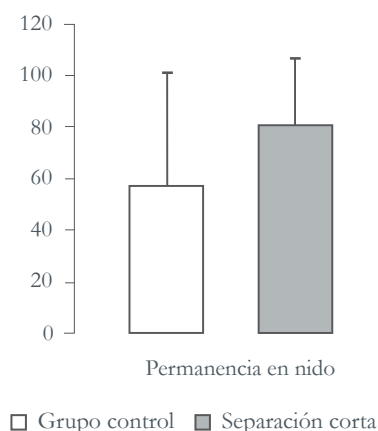
Figura 2. Tiempo en minutos promedio de la conducta de cuidado materno: permanencia en el nido. Hembras: control □ ( n = 7 ) y separadas ■ ( n = 7 ). No se encontraron diferencias significativas aplicando una prueba t .
