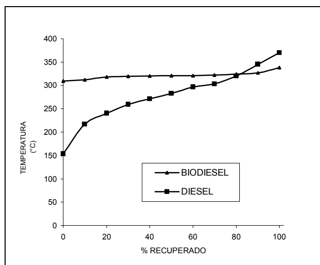
Figura 1. Curvas de destilación combustibles utilizados.
