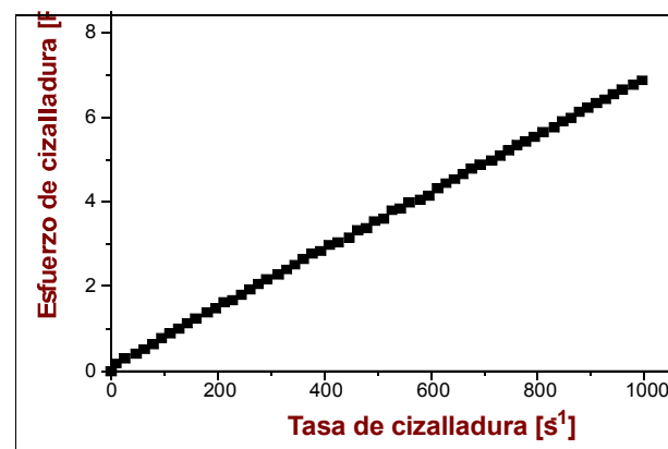
Figura 2. Reograma del BACP a 24°C.
