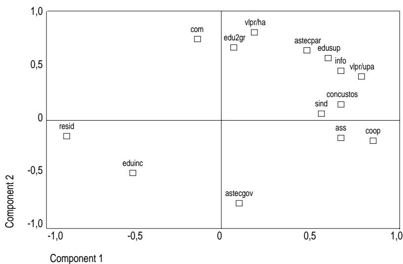
Figura 1. Resultado gráfico del análisis multivariado, extraídos dos componentes principales, después de la rotación por el método Varimax
