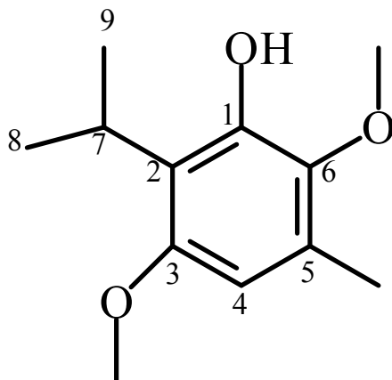
Figura 1. Estructura del Isoespintanol
