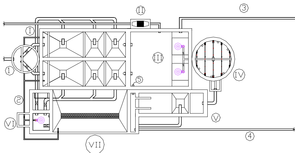
Fig. 5. Vista superior de la planta para el tratamiento de las aguas residuales de formas terminadas del Laboratorio "Julio Trigo". I Tanque séptico. II Cámara de rejillas. III Depósito de bombeo. IV Filtro biológico. V Sedimentador. VI Foso de lodos. VII Lechos de secados de lodo. 1 Registro de entrada al tanque séptico y caja de válvulas. 2 Caja de válvulas del foso de lodos. 3 By pass. 4 Emisario hacia el río. 5 Recirculación.
