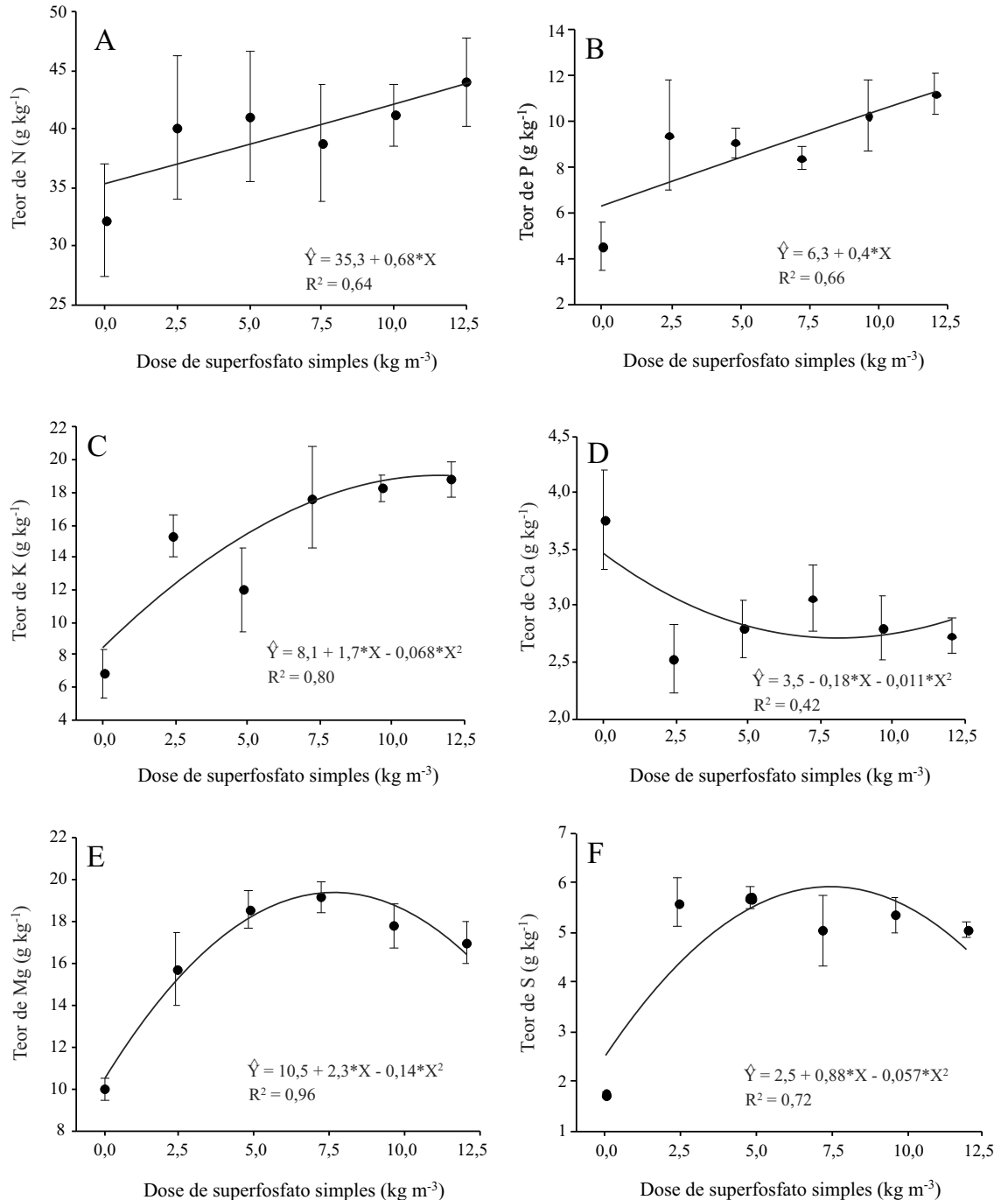
Figura 2 - Efeito de doses de superfosfato simples sobre os teores de nitrogênio (A), fósforo (B), potássio (C), cálcio (D), magnésio (E) e enxofre (F) na parte aérea de plântulas de pinhão manso. Barras verticais indicam o desvio padrão da média
