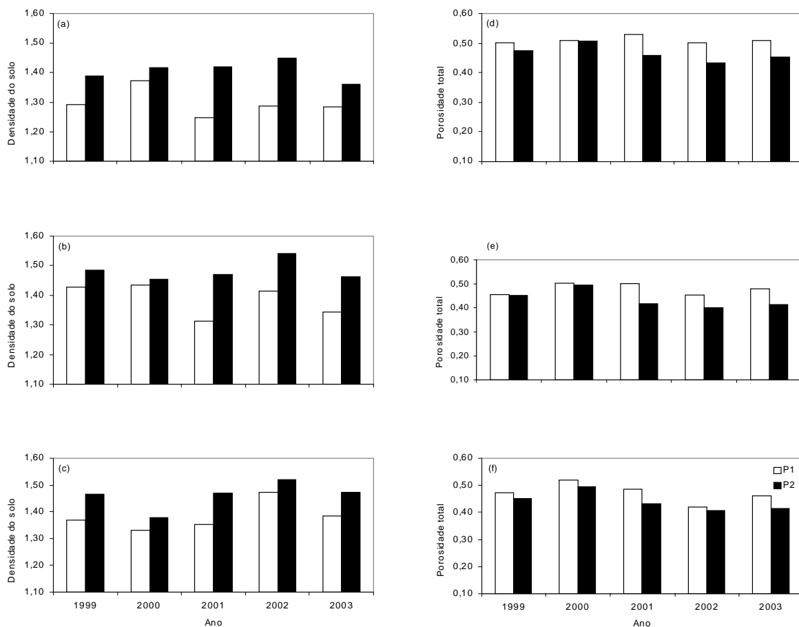
Figura 1. Valores médios da densidade do solo ( \text{Mg m}^{-3} ) e da porosidade total ( \text{m}^3 \text{m}^{-3} ), obtidos em dois sistemas de manejo do solo (P1: plantio direto seguido anualmente de um preparo com arado; P2: plantio direto contínuo), quatro sistemas de rotação de culturas e cinco anos de cultivo, nas camadas 0-10 cm (a, d), 10-20 cm (b, e) e 20-30 cm (c, f) de profundidade (Santo Antônio de Goiás, GO 2004).
