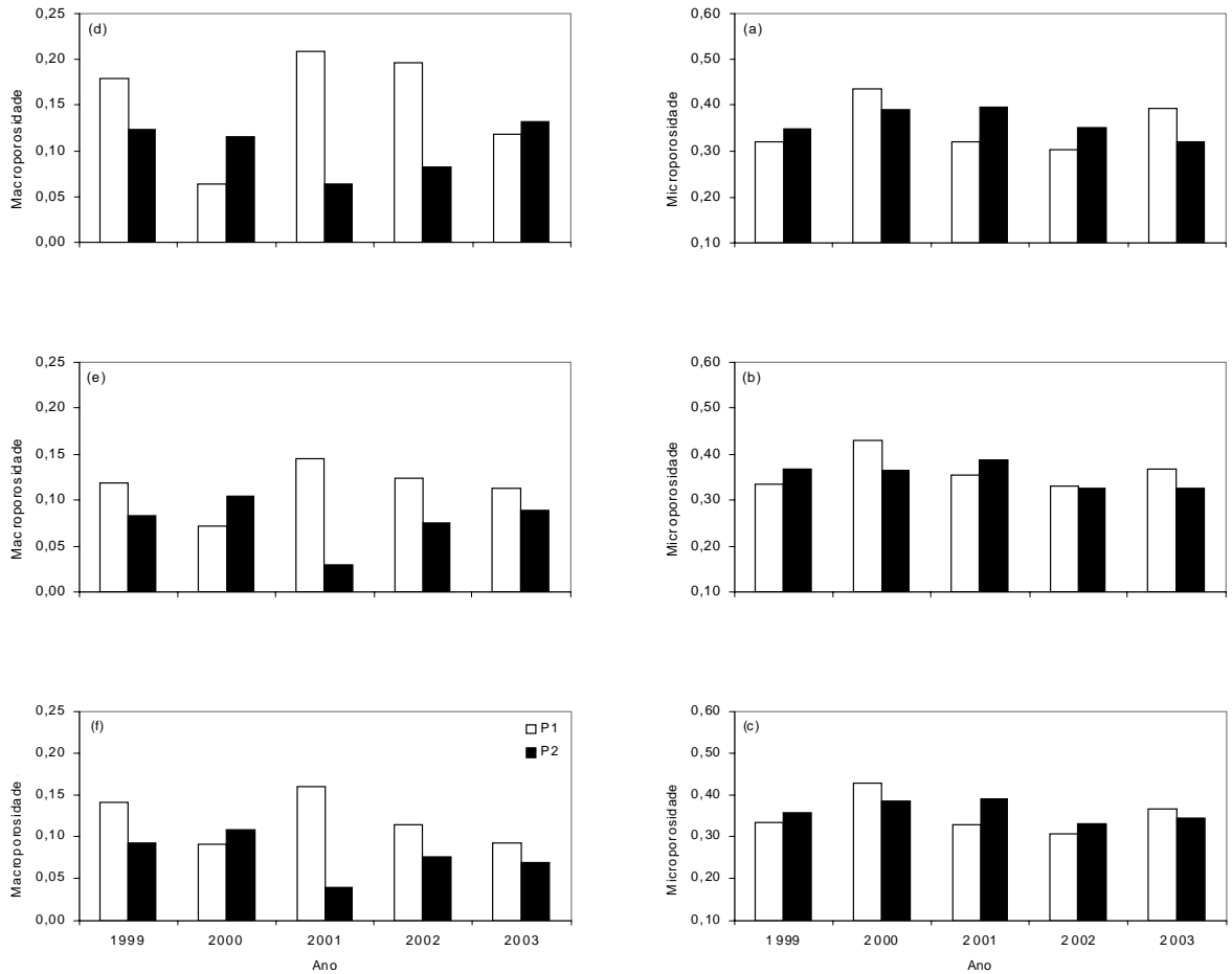
Figura 2. Valores médios da microporosidade e da macroporosidade, em m^3 m^{-3} , obtidos em dois sistemas de manejo do solo (P1: plantio direto seguido anualmente de um preparo com arado; P2: plantio direto contínuo), quatro sistemas de rotação de culturas e cinco anos de cultivo, nas camadas 0-10 cm (a, d), 10-20 cm (b, e) e 20-30 cm (c, f) de profundidade (Santo Antônio de Goiás, GO 2004).
