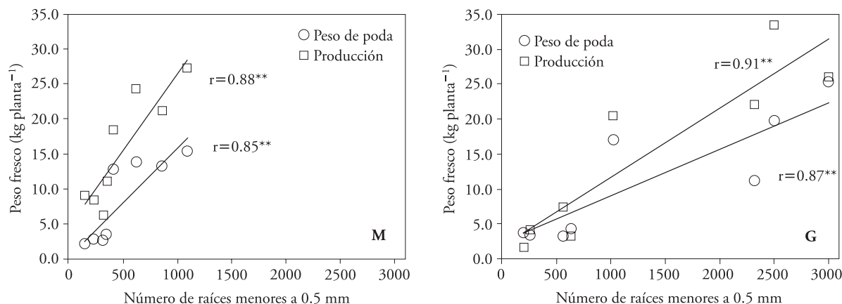
Figura 2. Relación lineal entre el número de raíces menores a 0.5 mm y el peso de poda y producción por planta (como peso fresco), para calicatas de 1.2×1.2 m en suelo de texturas media (M) y calicatas de 1.2×1.6 m suelo de texturas gruesas (G). (** Significativo, p \leq 0.01 ).
