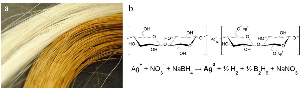
Figura 2. a. Comparación de la coloración de las fibras limpias (blanco) y las fibras modificadas con nanopartículas de plata (dorado). b. Reacción durante la síntesis de NPs de Ag sobre fibras de fique.
