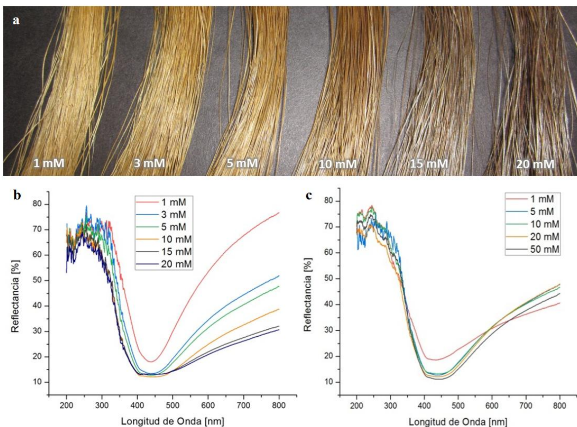
Figura 3. a. Fotografía de las fibras de fique modificadas con NPs de Ag variando la concentración de AgNO 3 . b. Espectros de reflectancia difusa variando la concentración de AgNO 3 . c. Espectros de reflectancia difusa variando la concentración de NaBH 4 .
