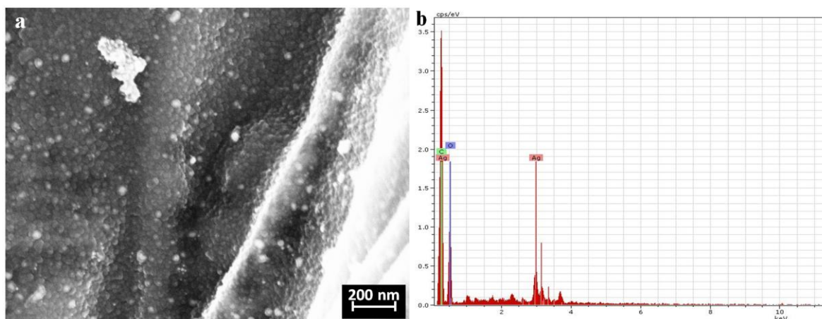
Figura 4. a. Micrografía SEM de las fibras modificadas con Ag NPs utilizando condiciones óptimas de síntesis. b. Espectro EDX de las fibras modificadas con Ag NPs utilizando condiciones óptimas de síntesis.
