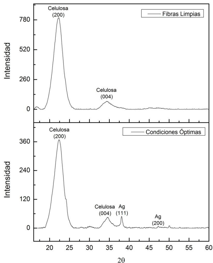
Figura 4. Difractogramas de las fibras de fique limpias y los bionanocompositos de fibras de fique y nanopartículas de plata sintetizados con condiciones óptimas.
