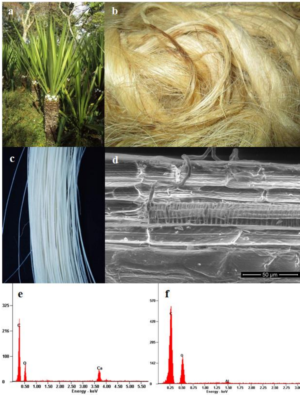
Figura 1. a. Planta de Fique. b. Fibras de fiquesin tratamiento. c. Fibras de fique limpias. d. Micrografía de una fibra de fique. e. Espectro EDX de las fibras de fique crudas. f. Espectro EDX de las fibras de fique limpias.
