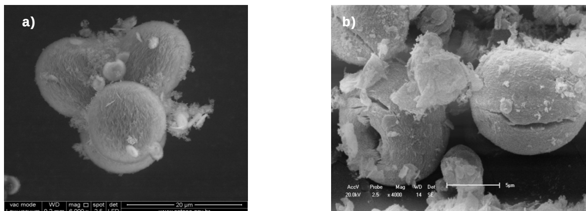
Fig. 3: Micrografías de la zeolita MCM-22 obtenidas por el método de síntesis hidrotermal (método A) y las obtenidas por el método B.
