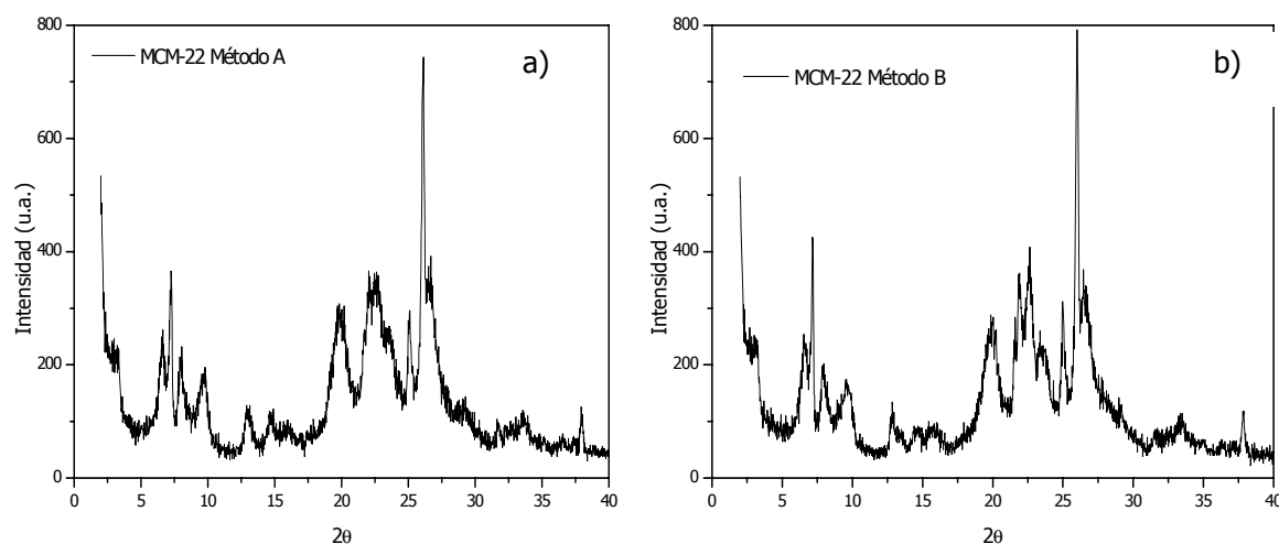
Fig. 2: Los patrones de difracción de rayos X de la zeolita MCM-22 obtenidos a partir de la síntesis hidrotermal. a) método A y b) el método B.
