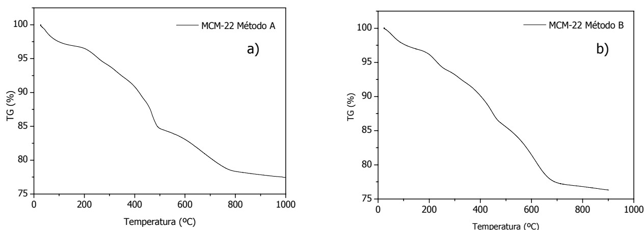
Fig. 4: TG curvas de la zeolita MCM-22 obtenidas por síntesis hidrotermal a) método A y b) método B.
