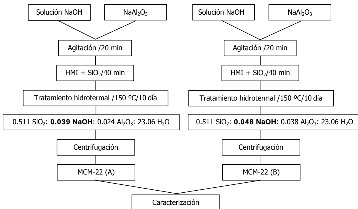
Fig. 1: Diagrama de las etapas de preparación de la zeolita MCM-22 (métodos A y B).
