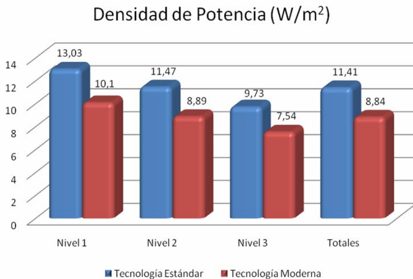
Gráfico 2. De densidad de potencia por metro cuadrado de local.
