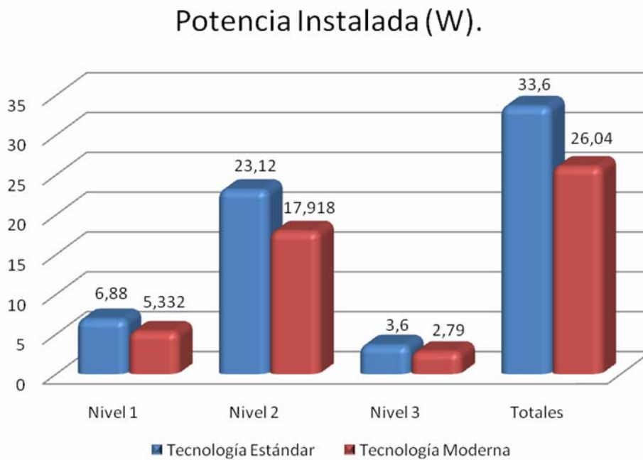
Gráfico .1. De potencia activa instalada por cada nivel de la edificación.
