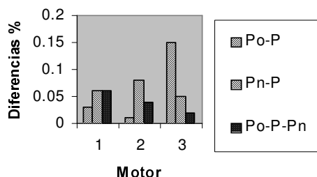
Diferencias comparativas de los motores.
