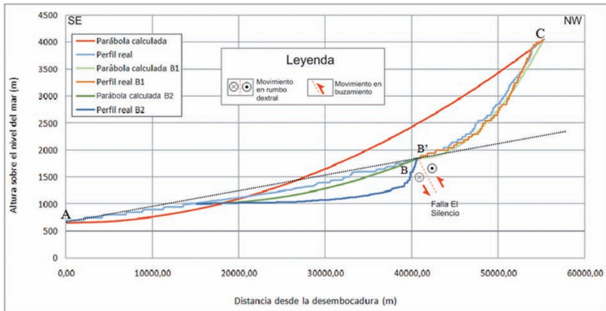
FIGURA 27. Perfil longitudinal fluvial y parábola teórica obtenida para la cuenca del río Combeima. Se presentan las relaciones obtenidas entre las parábolas calculadas B1 (bloque NW) y B2 (bloque SW) y sus perfiles reales, que reafirman la cinemática inversa de la Falla El Silencio.
