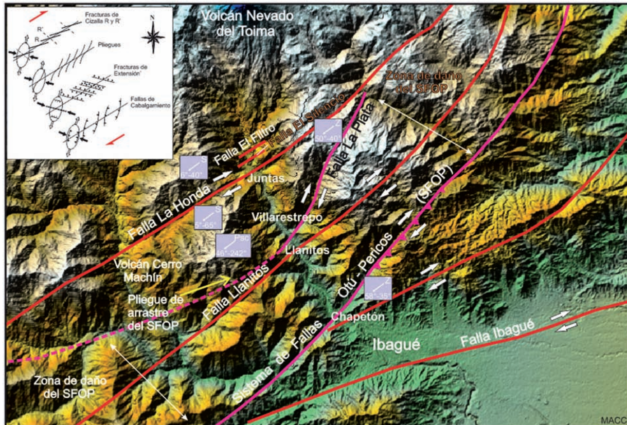
FIGURA 2. Estilo estructural propuesto para la cuenca del río Combeima. En el recuadro se esquematiza la orientación teórica de fallas y pliegues en una zona rumbo deslizante dextral.
