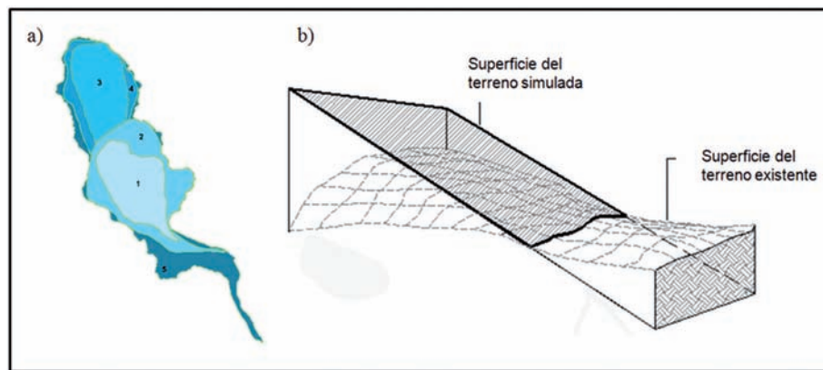
FIGURA 3. (a) Etapas evolutivas sugeridas, para la evaluación del proceso de erosión remontante en la zona de estudio. (b) Bloque diagrama donde se presenta las superficies: actual y superior (“tapa”) empleadas para el cálculo del volumen desplazado durante estas fases.
