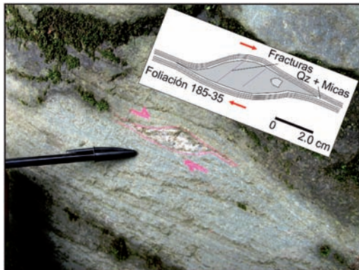
FIGURA 14. Indicador cinemático en forma de “pez”, con desarrollo de colas (Qz + micas) a partir de un núcleo rígido de cuarzo (Qz), con cinemática de tipo dextral en rocas asociadas al Complejo Cajamarca, aflorantes en la quebrada “Gonza” (González).
