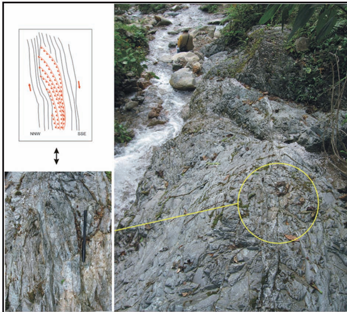
FIGURA 6. Estructuras tipo Pop Up , rasgo relacionado con la actividad tectónica del Sistema de Fallas Otú – Pericos, estructura ubicada en el cauce de la quebrada Cay. En el círculo amarillo terminación en cola de caballo inversa con cinemática dextral.
