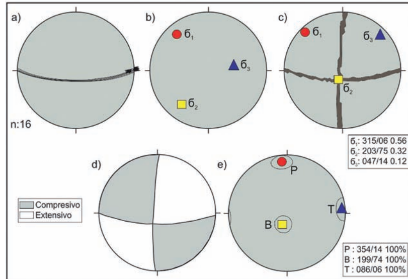
FIGURA 13. (a) y (b) Diagramas de esfuerzos resultante de la inversión de estrías medidas en la Falla La Honda (sector de la Virgen, aledaño al Corregimiento de Juntas). (c) Diagrama de diedros rectos calculado con base al desarrollo de Angelier et Mechler (1977). (d) Representación con sombras del diedro recto. (e) Diagrama de dispersión de ejes P y T.
