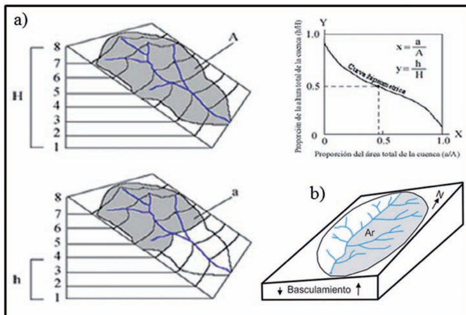
FIGURA 4. (a) Curva hipsométrica y (b) Factor de asimetría (FA) de la cuenca de drenaje, modificado de Keller and Pinter (1996).
