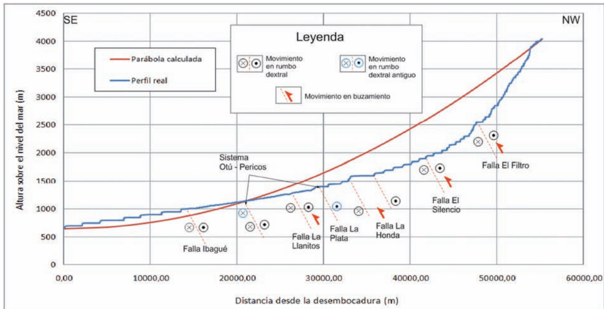
FIGURA 26. Perfil longitudinal fluvial y parábola teórica obtenida para la cuenca del río Combeima. Se observa a la altura del Sistema de Fallas Otú-Pericos un punto de inflexión de la cuenca, el cual puede ser relacionado con la depositación del Abanico de Ibagué y la actividad tectónica de las fallas en este tramo de la cuenca.
