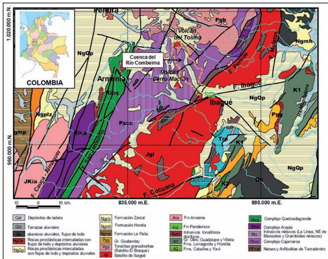
FIGURA 1. Mapa geológico generalizado de la zona de Falla Ibagué, departamentos de Tolima, Quindío y Valle del Cauca. Tomado de INGEOMINAS (1997).
