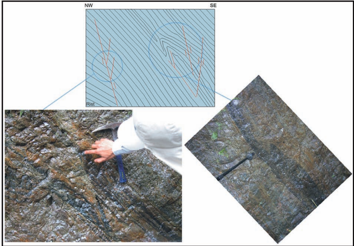
FIGURA 7. Fallas de tipo inverso con levantamiento SSE sobre NNW y pliegues por propagación de falla asociados a sistemas de abanicos imbricados. Sector La Cascada, quebrada afluente a la quebrada Cay.
