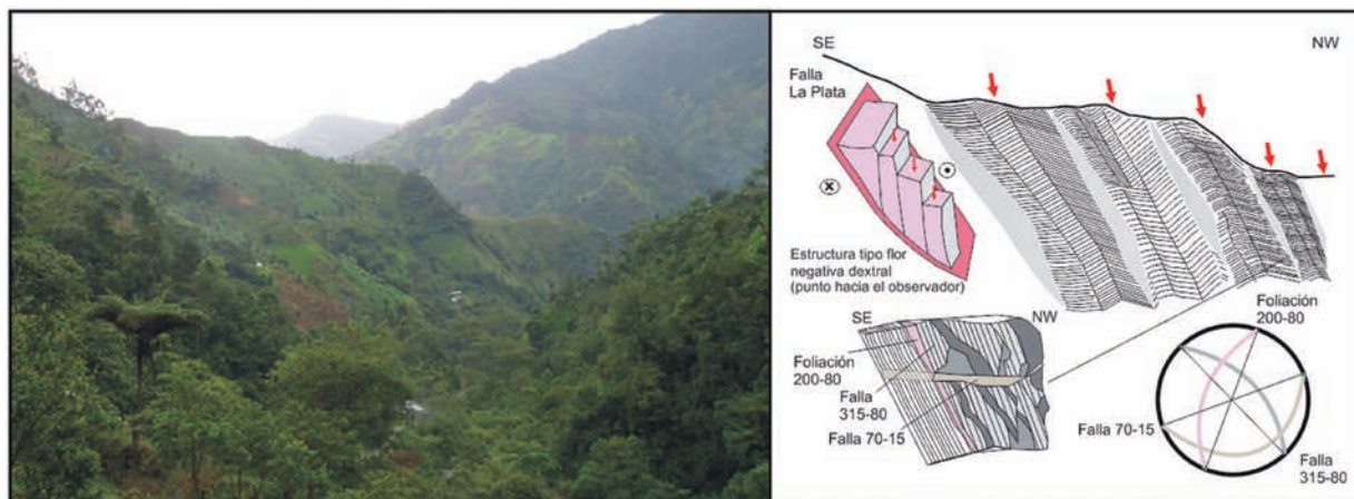
FIGURA 20. Sistemas extensionales asociados a fallas de tipo normal, que involucran bloques de gran dimensión en respuesta a los fenómenos de compensación del transporte tectónico. Margen derecha quebrada La Plata, vereda Pico de Oro.
