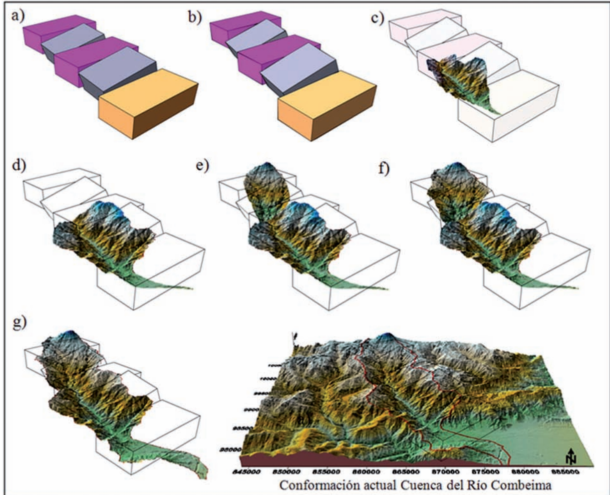
FIGURA 24. Proceso de erosión remontante o regresiva, donde se identifican como mínimo cinco etapas de desarrollo hasta la conformación actual la cuenca del río Combeima y su íntima relación con el estilo estructural propuesto. (a) y (b) Fases tectónicas, (c) Primera etapa evolutiva, (d) Segunda etapa evolutiva, (e) Tercera etapa evolutiva, (f) Cuarta etapa evolutiva, (g) Quinta etapa evolutiva y conformación actual de la cuenca.
