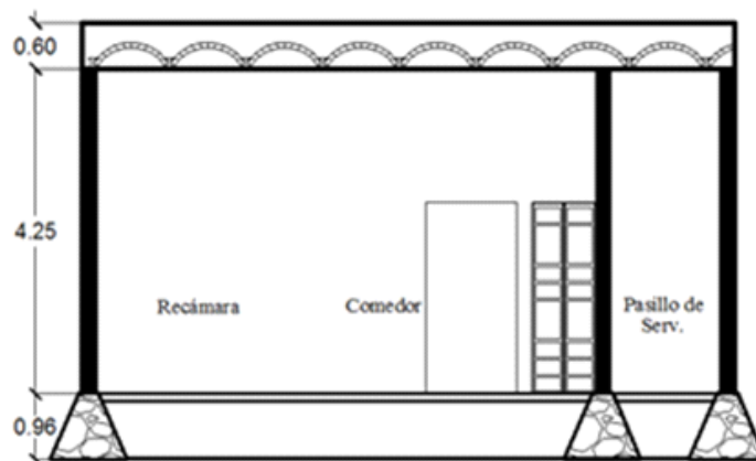
Figura N° 8. Corte transversal A-A'
