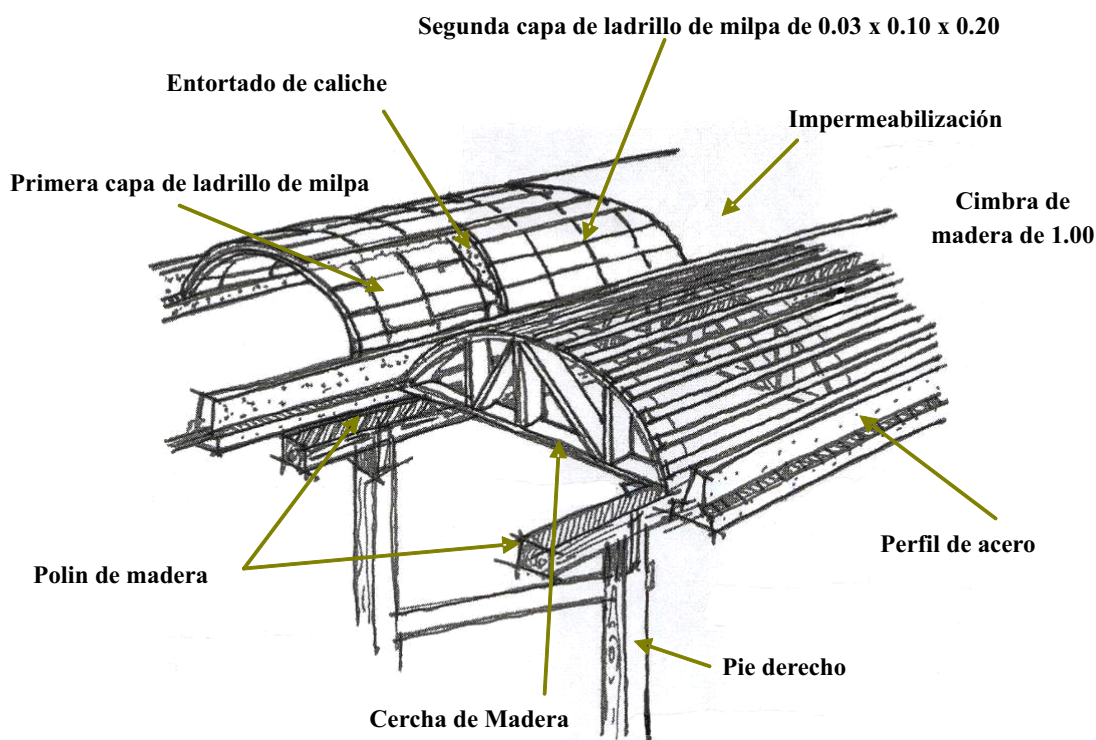
Figura N° 5. Boceto de detalle de bóveda curva o catalana de la Vivienda tradicional
