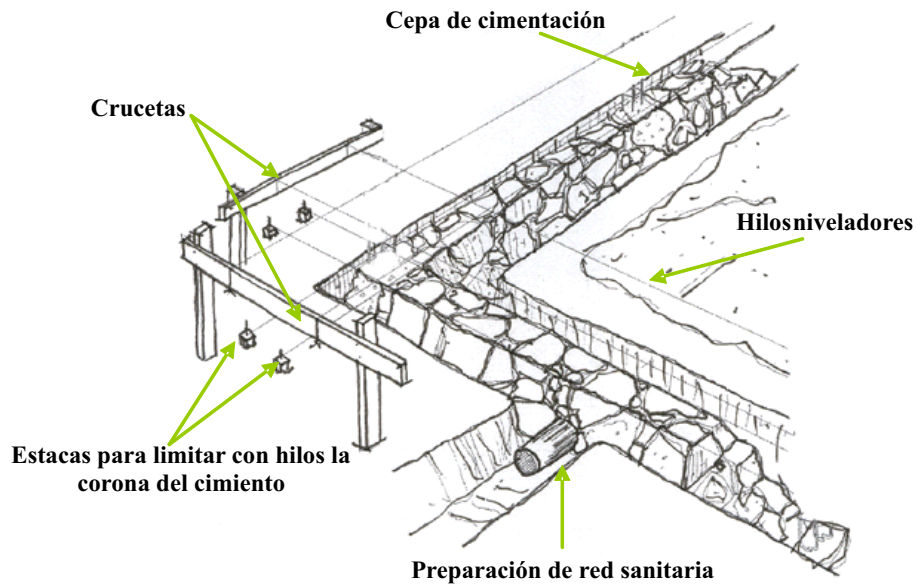
Figura N° 2. Boceto de cimientos corridos de la vivienda tradicional
