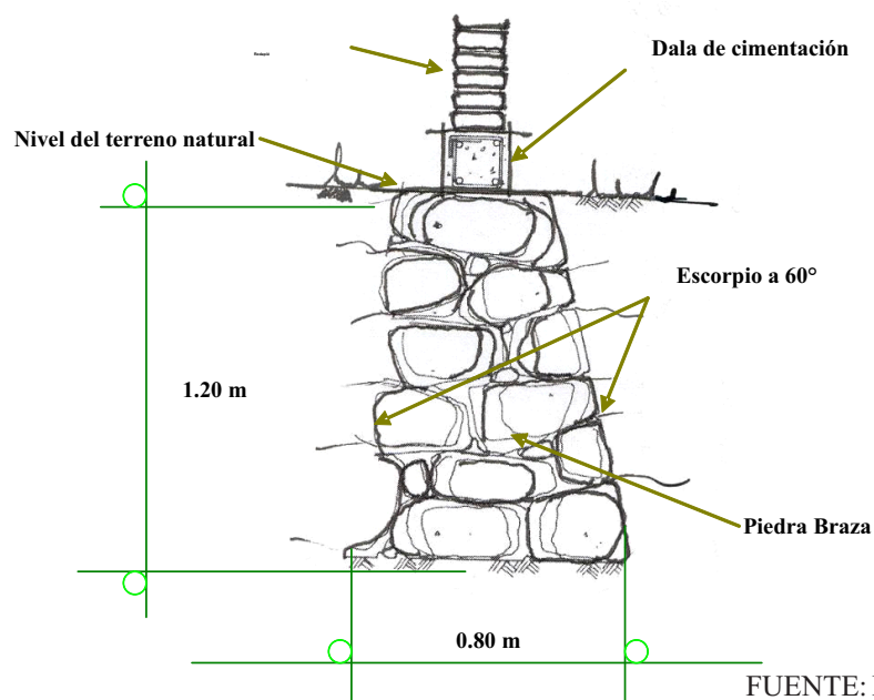
Figura N° 3. Boceto de cimiento de piedra braza de la vivienda tradicional
