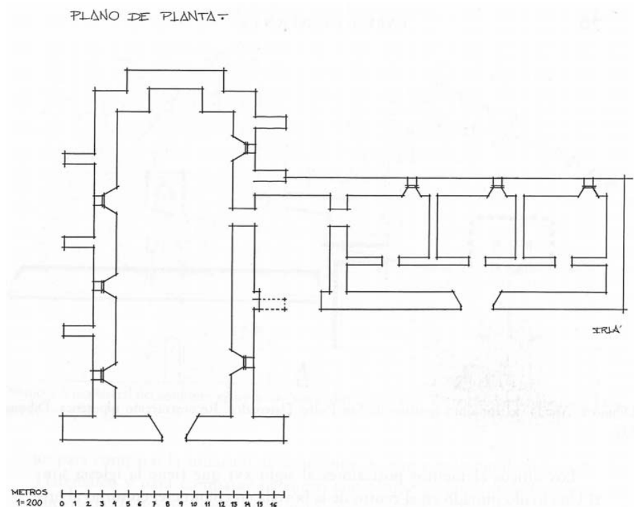
Dibujo 1. Planta del conjunto agustino de San Pedro Tlatemalco. Reconstrucción hipotética. Dibujo: Irla Granillo.
