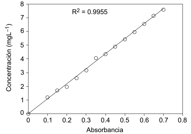
Fig. 3. Curva de calibración para la cuantificación de azul 1
