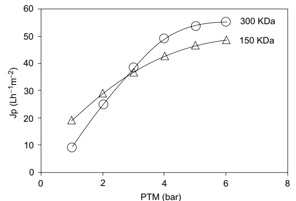
Fig. 4. Flujo de permeado ( J_p ) del agua desionizada en función de la PTM
