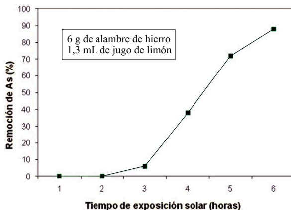
Figura 4. Grado de remoción del arsénico en función del tiempo.
