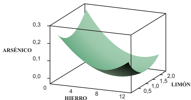
Figura 3. Superficie de respuesta de arsénico vs limón y hierro.
