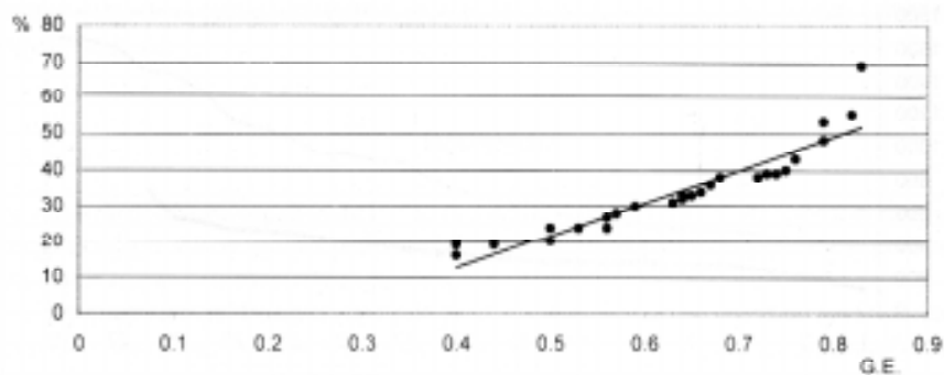
Fig. 5. Correlación entre gravedad específica y grosor de pared de fibras en las especies del bosque mesófilo.
