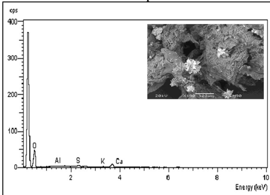
Figura 6. MEB del biomaterial antes del tiempo de contacto
