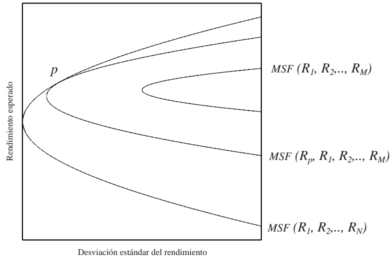
Gráfica 1 Ilustración de la proposición 1
