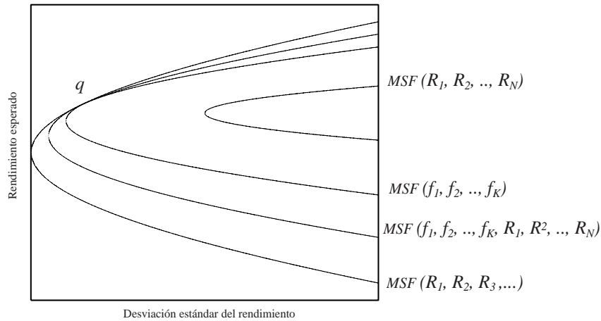
Gráfica 2 Ilustración de la proposición 2
