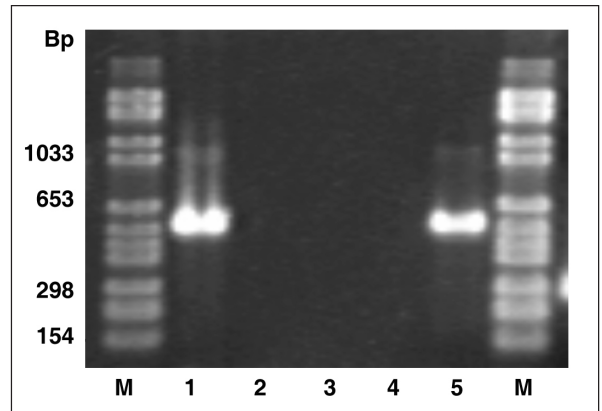
FIGURA 3. Amplificados de los genes que codifican la resistencia de estaphylococcica a meticilina ( mecA ) de S. aureus con un tamaño de 530 pb (carril 1: cepa positiva a mecA cepa de campo de Brasil) carriles 2-4: cepas negativas, carril 5: control positivo M: marcador de peso molecular del ADN (Serva DNA standard pBR328Mix, Heidelberg, Germany).
