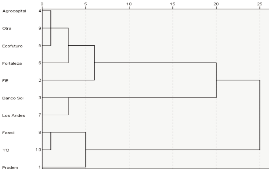
Figura 2 Dendograma Análisis Cluster Jerárquico
