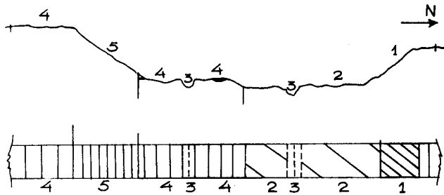
Figura 2. Parada 2: perfil de un área quebrada
