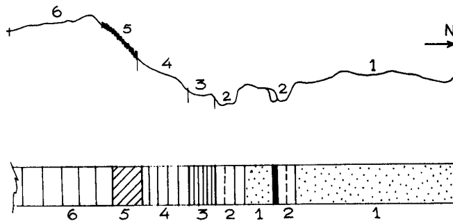
Figura 3. Parada 3: perfil del Cerro Petaca
