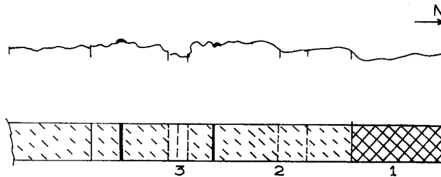
Figura 1. Parada 1: perfil de un área antropizada 1-ripiera: con vegetación esporádica o accidental. 2-basural: con vegetación ruderal de plantas exóticas de jardines, cultivos, etc. 3-cauce: con vegetación riparia y del álveo representadas por Proustia cuneifolia y Phacelia artemisioides .
