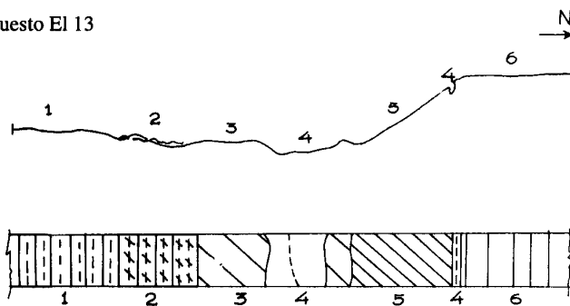
Figura 4. Parada 4: perfil del área en proximidades. de la Cancha
