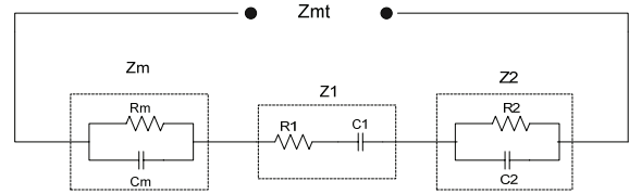
Figura 5 Esquema del circuito utilizado para obtener la impedancia de los tejidos. Con Z_m : impedancia de la muestra; Z1 : impedancia medida de los electrodos; Z2 : impedancia comercial conectada en serie y Z_{mt} : impedancia total medida
