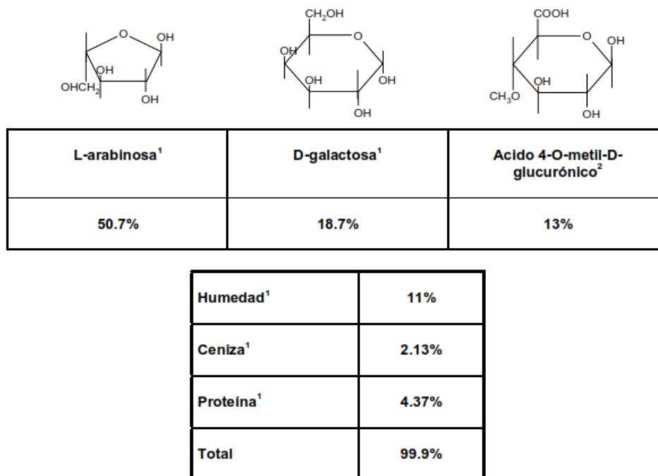
Figura 4.- Componentes de la goma de mezquite (Aspinall y Whitehead, 1970).
