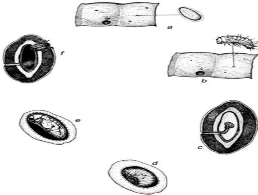
Figura 5.- Reconstrucción del ciclo vital de los brúcidos en las vainas de Prosopis : a. huevos pegados a la superficie de la vaina o depositados en las grietas de la vaina o en los foros de salida de un brugo adulto (orificio redondo). b. orificio de entrada de la primera etapa de la larva que ha perforado la pared de la vaina, y primera etapa larval, agrandada, para mostrar los pelos, espinas y patas modificadas para entrar en la semilla. c. corte transversal de la vaina y de la semilla para indicar el hueco hecho por la primera fase larval al entrar. d. fase posterior de la larva, dentro de la cavidad roída en la semilla. e. pupa dentro de la cámara de alimentación larval. f. adulto saliendo a través del orificio, perforado por la última fase larval.
