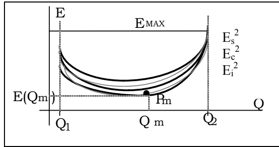
Figura 5. Nuevo haz borroso que cumple las restricciones
