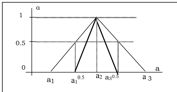
Figura 3. Números borrosos triangulares de soporte reducido
