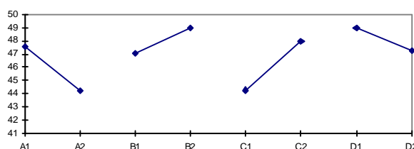
Fig. 4. ANOVA. Criterio "mayor-mejor". Variable A (longitud de onda) a nivel 1; Variable B (Volumen de HCl conc. a adicionar) a nivel 2; Variable C (Tiempo de calentamiento) a nivel 2 y Variable D (Volumen de aforo de los estándares) a nivel 1.
