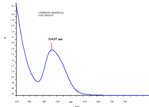
Fig. 3. Espectro visible del complejo coloreado.
