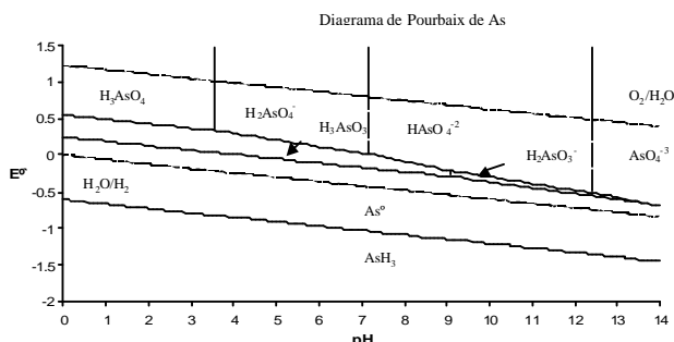
Fig. 1. Diagrama de Pourbaix para el arsénico
