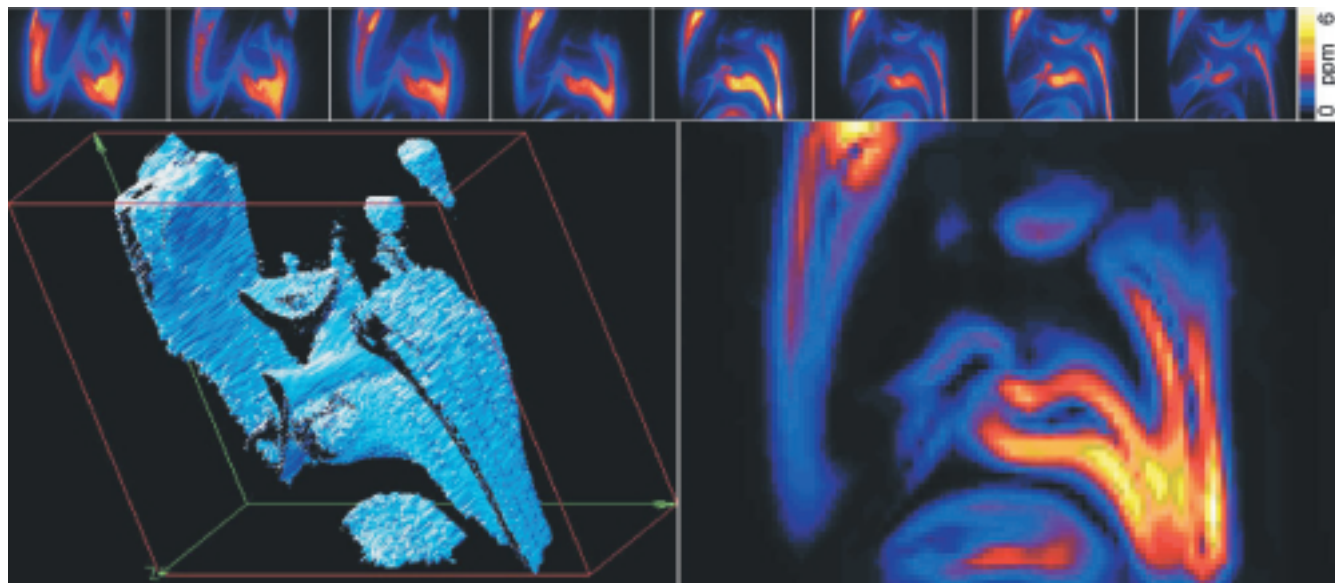
Imagen tridimensional de la fracción volumétrica de hollín en una llama de difusión turbulenta. Arriba: ocho cortes bidimensionales a través de la llama. Abajo izquierda: superficie de isoconcentración de 1 ppm. Abajo derecha: gradiente de concentración de hollín tridimensional
