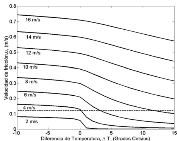
Figura 4. Comportamiento de la velocidad de fricción del viento en función de la diferencia de temperatura de aire-mar ( ^\circ\text{C} ). Los valores negativos representan inestabilidad, mientras los valores positivos representan condiciones estables. El cero representa condiciones de estabilidad neutra.
