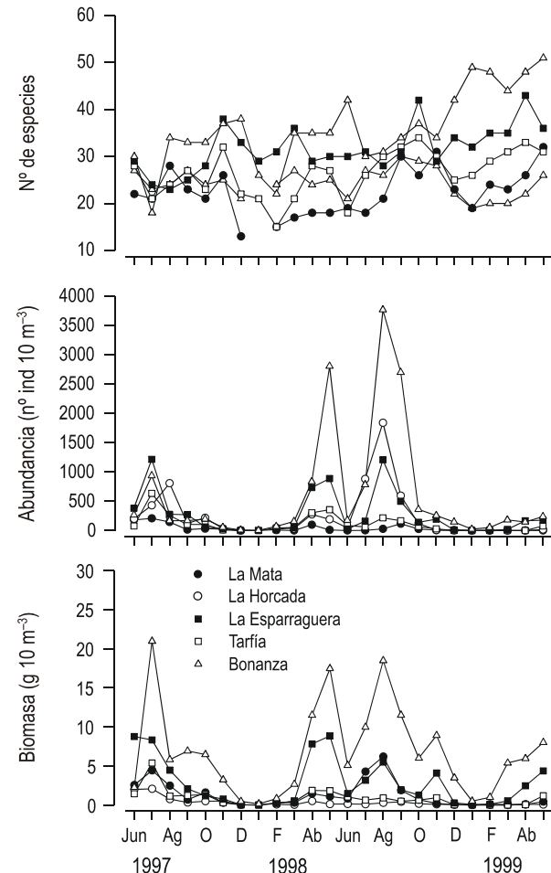
Figura 3. Evolución mensual del número de especies, de la abundancia y de la biomasa de la macrofauna acuática en las cinco estaciones de muestreo.
