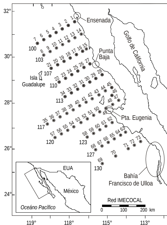
Figura 1. Red de estaciones del programa Investigaciones Mexicanas de la Corriente de California (IMECOCAL). Los números enteros corresponden a la línea hidrográfica y los decimales a la estación.
