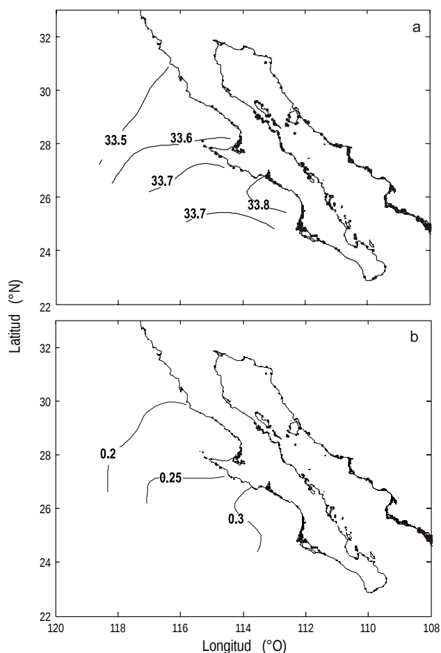
Figura 4. Salinidad de la superficie de 25\sigma_\theta : (a) promedio y (b) desviación estándar.
