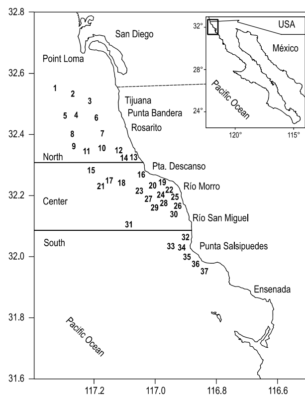
Figura 1. Área de estudio y estaciones de muestreo de sedimentos superficiales en las zonas norte, centro y sur de la costa noroccidental de Baja California (agosto de 1998).
