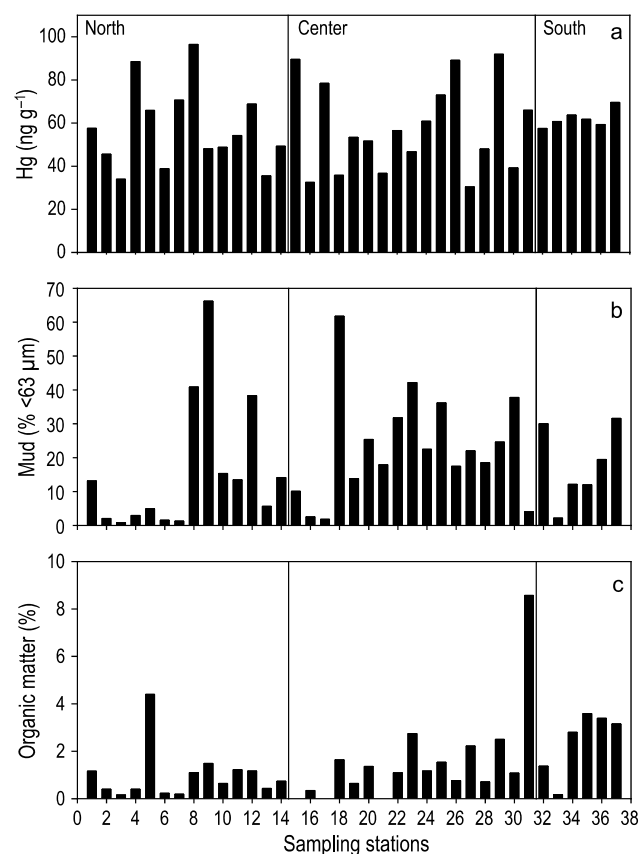
Figura 2. Distribución espacial de Hg, lodos y materia orgánica en la costa noroccidental de Baja California (agosto de 1998).
