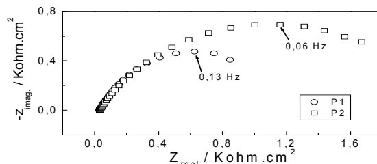
Figura 8. Impedancia de acero al carbono desnudo (P1-P2) en solución 0,2 M de \text{Na}_2\text{SO}_4
