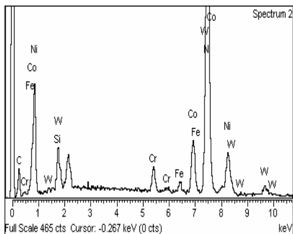
Figura 1. Espectro de EDS de los polvos Metaceram 29123, para la capa intermedia de los recubrimientos
