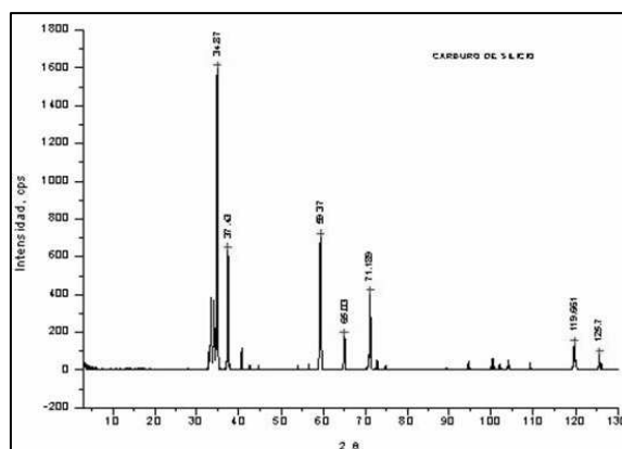
Figura 2. Difractograma del polvo de SiC usado para la capa final de los recubrimientos tricapas Figure 2. DRX pattern of the SiC powder used to deposit the layer of-the tri-layered coatings
