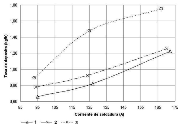
Figura 2. Comportamiento de la tasa de deposición con la variación de corriente de soldadura.
