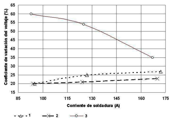
Figura 4. Comportamiento del coeficiente de variación del voltaje con la variación de la corriente de soldadura.
