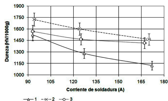
Figura 5. Comportamiento de la dureza promedio del depósito con la variación de la corriente de soldadura.
