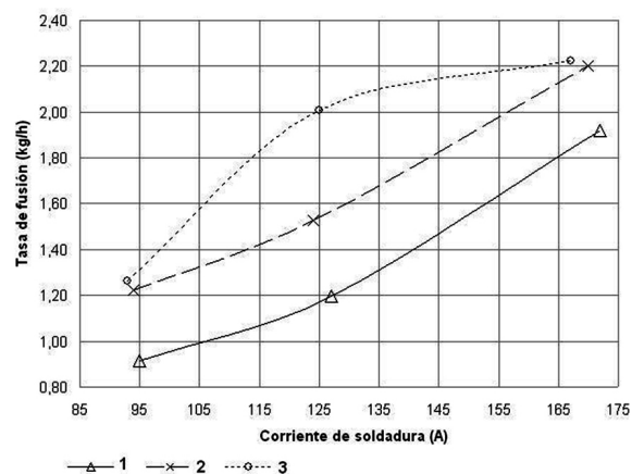
Figura 1. Comportamiento de la tasa de fusión con la variación de la corriente de soldadura.
