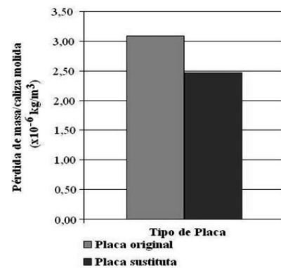
Figura 7. Pérdida de masa de las muestras para 16200 m 3 de roca caliza molida.
