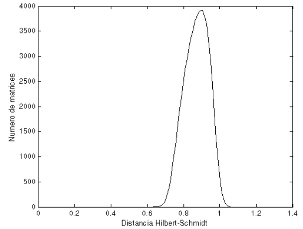
FIGURA 2. Histograma del número medio de matrices seudopuras extendidas y entrelazadas que tienen una distancia de Hilbert-Schmidt dada al “estado gato”, considerando \epsilon = 5 \times 10^{-4} . Se generaron (aleatoriamente) 500,000 matrices en cada ciclo de cálculos y se realizó un promedio sobre 10 ciclos.
