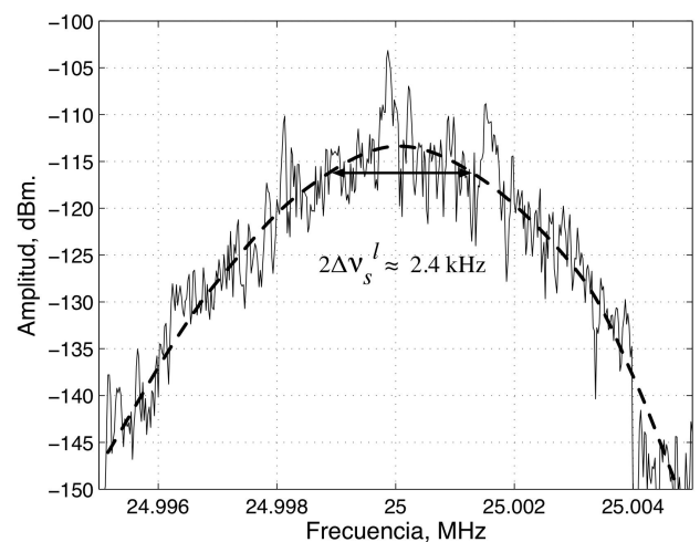
FIGURA 10. Espectro auto-heterodina retrasado de la emisión de Stokes del láser Brillouin.
