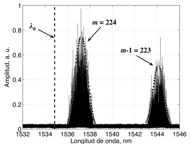
FIGURA 4. Señal de Stokes en el puerto D (Fig 1) al hacer un barrido de la longitud de onda del bombeo \lambda_p .
