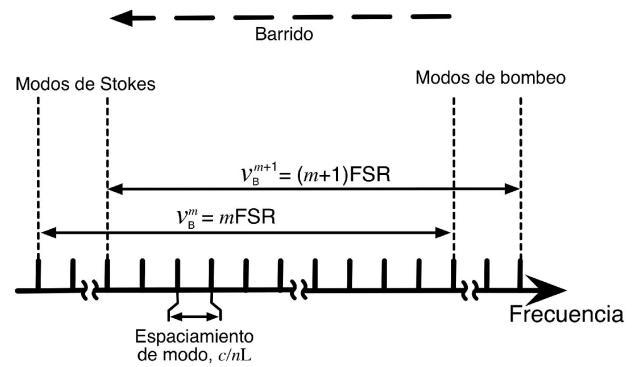
FIGURA 2. Condiciones para lograr la doble resonancia dentro de la cavidad.
