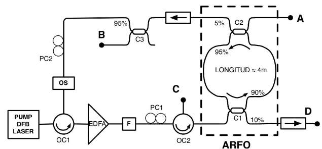
FIGURA 7. Esquema experimental del láser de Brillouin con la cavidad ajustada. F-filtro óptico, IO- interruptor óptico.
