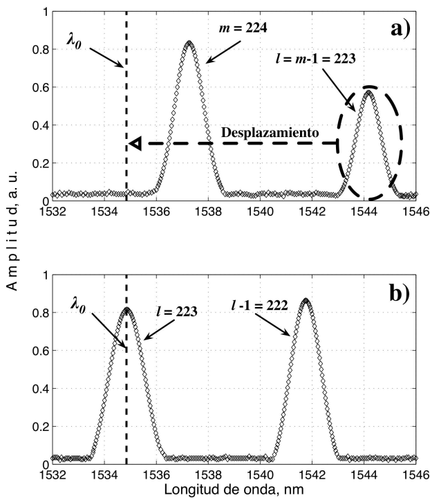
FIGURA 6. Aproximaciones gaussianas de la señal de Stokes; a) cavidad no ajustada, b) cavidad ajustada.
