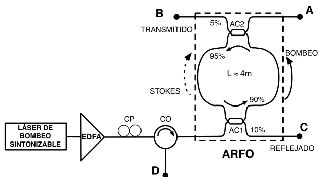
FIGURA 1. Esquema experimental para observar la doble resonancia. ARFO -anillo resonador de fibra óptica, CP- controlador de polarización, CO -circulador óptico, AC1 y AC2- acoplador óptico.
