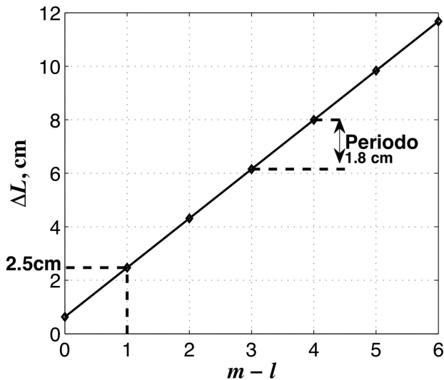
FIGURA 5. Longitud de corte de fibra en la cavidad \Delta L contra la diferencia entre el orden de los picos m-l .
