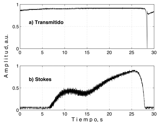
FIGURA 9. Trazos de osciloscopio de la señal de Stokes en doble resonancia; a) señal transmitida en el puerto B, y b) señal de Stokes en el puerto D.
