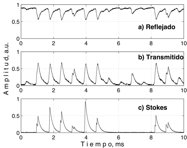
FIGURA 3. Trazos de osciloscopio de: a) señal reflejada registrada en el puerto C (Fig 1), b) señal transmitida en B, y c) señal de Stokes en D.
