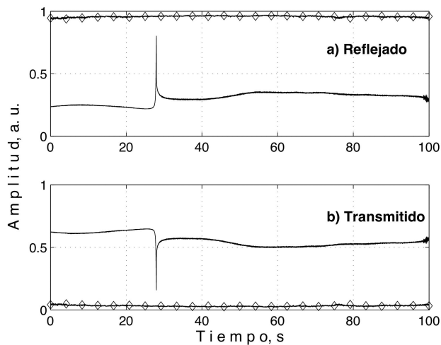
FIGURA 8. Trazos de osciloscopio del bombeo: a) reflejado en el puerto C, y b) transmitido en el puerto B; en línea continua con retroalimentación (-); en línea con marcas ( \diamond ) sin retroalimentación.
