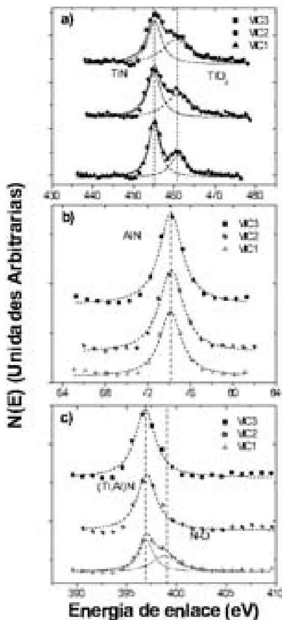
FIGURA 5. Espectros de energía de enlace obtenidos por espectroscopía electrónica para análisis químico de las películas MC1-MC3 en las regiones de Ti 2p, Al 2p, y N 1s.
