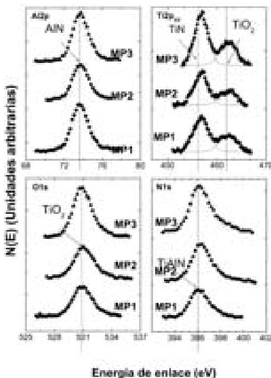
FIGURA 6. Espectros de energía de enlace obtenidas por espectroscopía electrónica para análisis químico de las películas MP1-MP3 en las regiones de Al 2p, Ti 2p, O 1s y N 1s.
