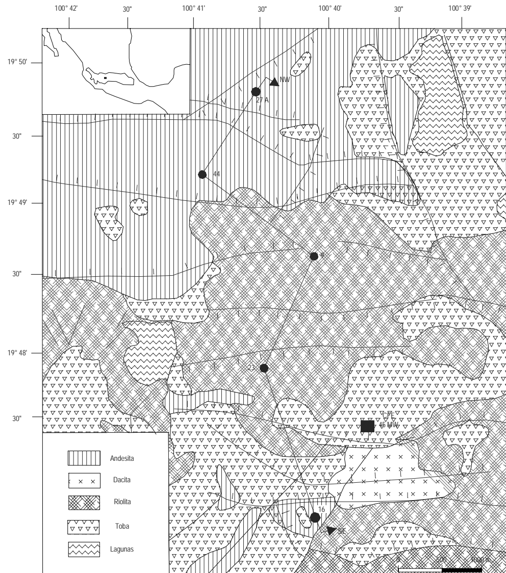
Figura 1.— Mapa geológico-estructural del campo geotérmico de Los Azufres, Mich. Se indica la posición de los pozos.
