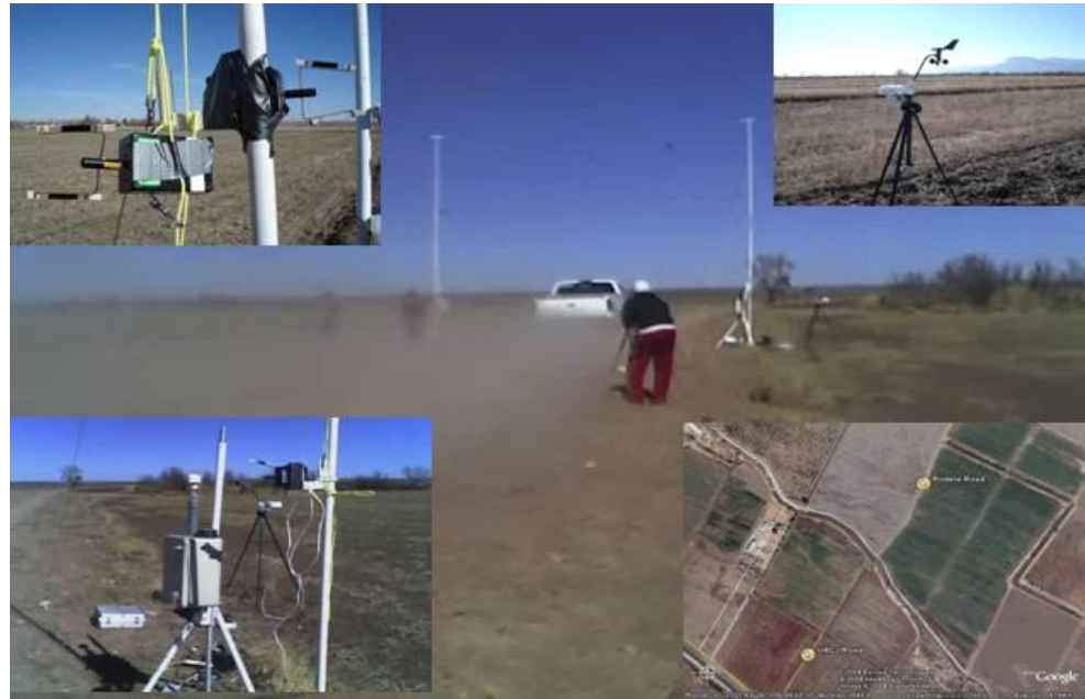
Figura 1. Rotores colgados de la torre (arriba izquierda), estación climática portátil (arriba derecha), muestreador de material particulado (MP) (abajo izquierda), foto de sitios experimentales Google (abajo derecha) y la camioneta corriendo por debajo de la torre y generando la nube de polvo en el camino no pavimentado del Valle de Juárez, Chihuahua, México.
