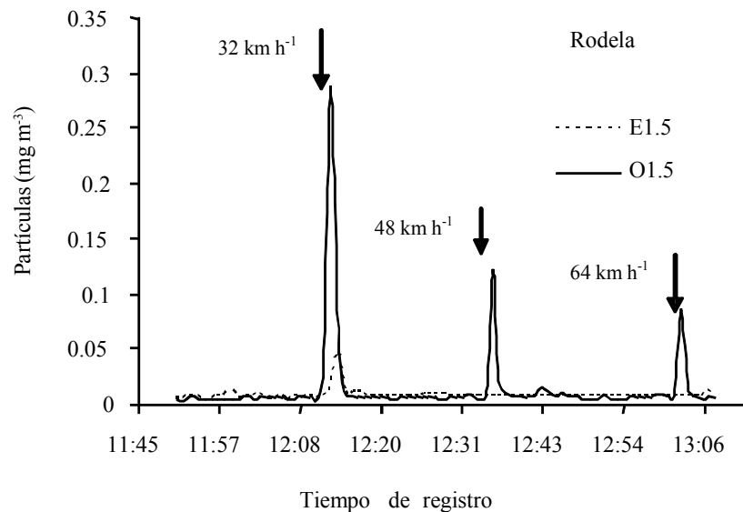
Figura 5. La cantidad de partículas (mg m -3 ) colectadas por el muestreador MET-1 ubicado al Este y Oeste de los caminos a 1.5 m sobre el nivel del terreno.
