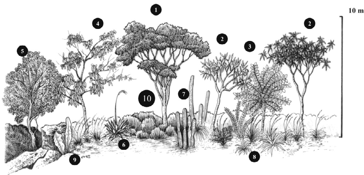
Figura 5. Perfil esquemático de la selva baja caducifolia. 1. Lysiloma acapulcense , 2. Plumeria rubra , 3. Comocladia engleriana , 4. Cochlospermum vitifolium , 5. Bursera cinerea , 6. Agave pendula , 7. Cephalocereus palmeri var. sartorianus , 8. Hechtia sp., 9. Anthurium schlechtendalii subsp. schlechtendalii , 10. Rhynchelytrum repens .
