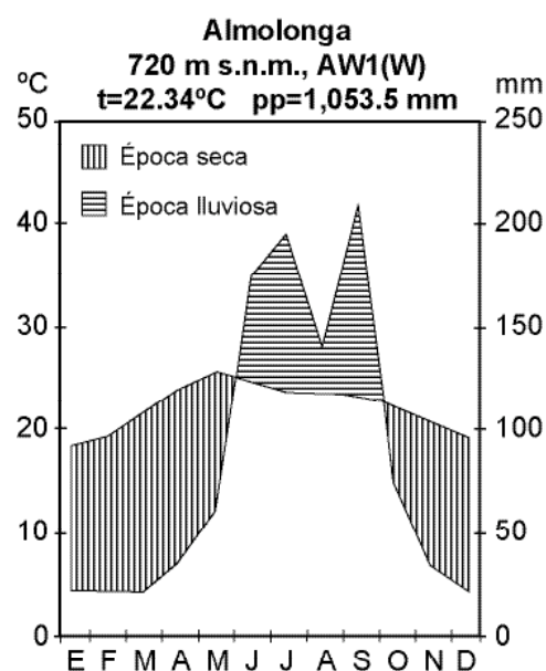
Figura 2. Diagrama ombrotérmico de Almolonga, Veracruz.
