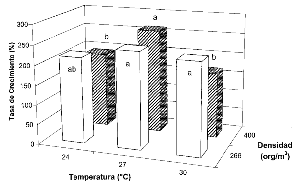
Figura 1. Efecto de la temperatura y la densidad de cultivo sobre la tasa de crecimiento en peso de juveniles de cabrilla arenosa cultivados en laboratorio.
