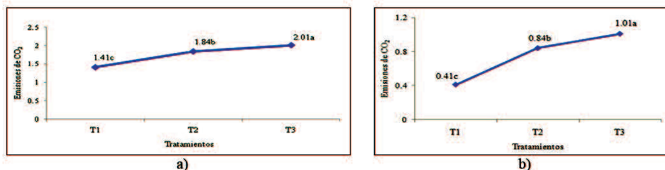
FIGURA 1. Relación salida/entrada de las emisiones y sostenibilidad de emisiones de CO 2 en los tres sistemas de laboreo comparados.
