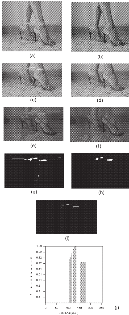
Fig. 7. Proceso de segmentación de la línea láser con una iluminación de 0 EV (valor de exposición estándar). (a) y (b) imágenes originales con y sin láser, respectivamente; (c) y (d) imágenes normalizadas con y sin láser, respectivamente; (e) y (f) sus correspondientes imágenes en canal rojo; (g) umbralización; (h) apertura; (i) centro de masa y (j) gráfica pixel-distancia.
