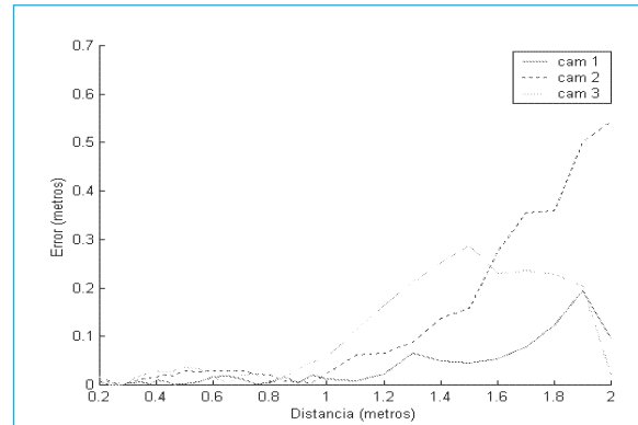
Fig. 4. Relación de error.
