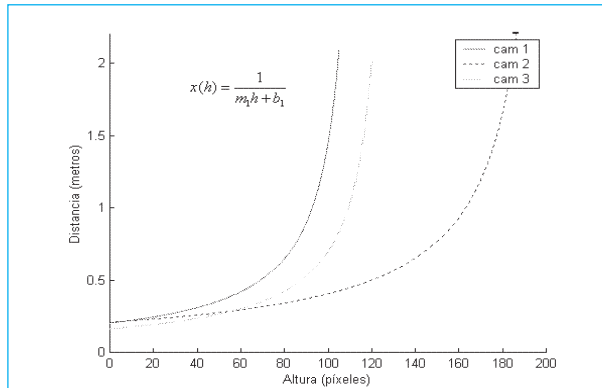
Fig. 2. Datos experimentales para los parámetros m_1 y b_1 .
