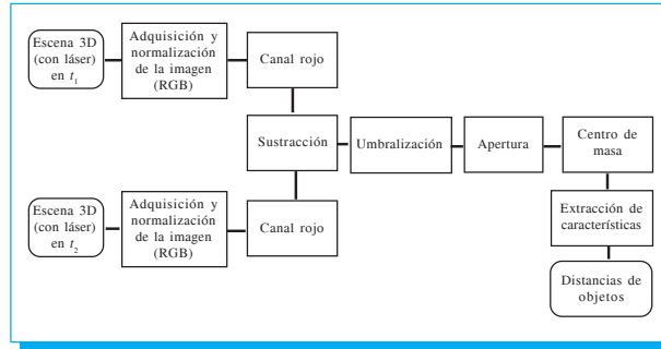
Fig. 5. Etapas de procesamiento de la imagen.
