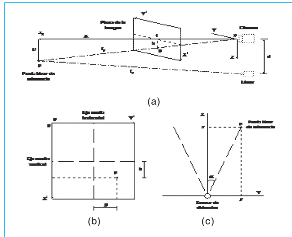
Fig. 1. Estimación de la posición de un objeto. (a) Vista de lado; (b) posición de un punto láser en la imagen de la cámara; (c) vista superior.
