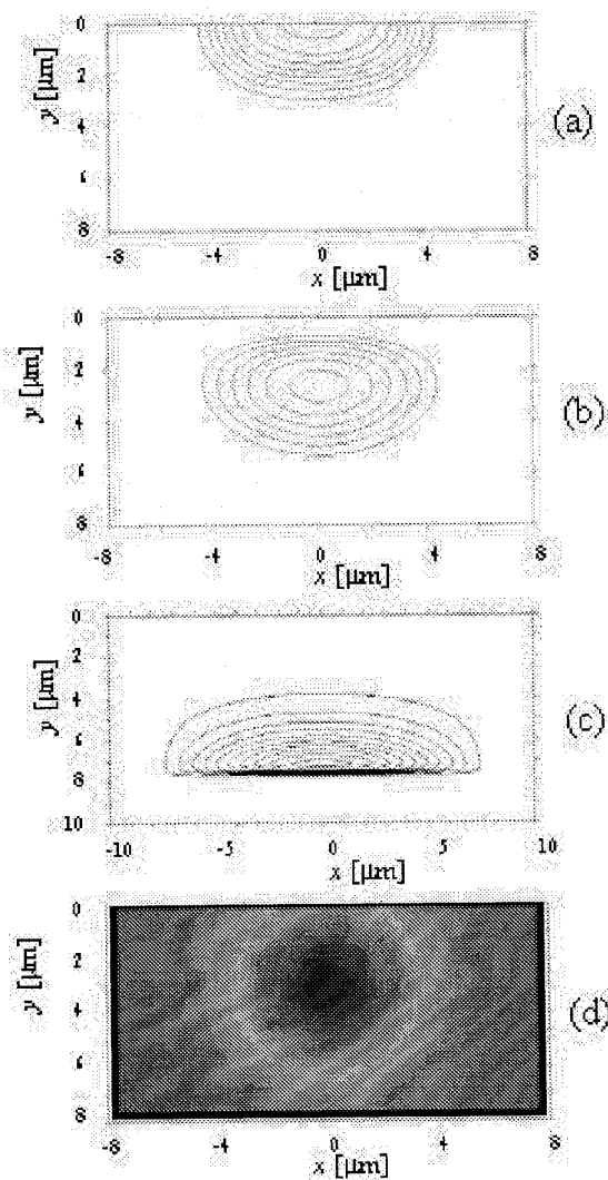
Figura 1: Representación gráfica de los perfiles de difusión, a) difusión primaria; b) difusión secundaria con baño de sales; c) difusión secundaria con baño de sales asistida por campo eléctrico y d) perfil de distribución de intensidad de luz que emerge de la guía de onda; x representa la posición lateral, la profundidad está representada por y .
