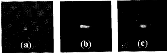
Figura 4: Modos que emergen de la guía de onda después de introducir luz láser. Las fotografías (a) y (b) representan el comportamiento modal para \lambda=632 nm; la fotografía (c) corresponde al comportamiento en \lambda = 1550 nm.
