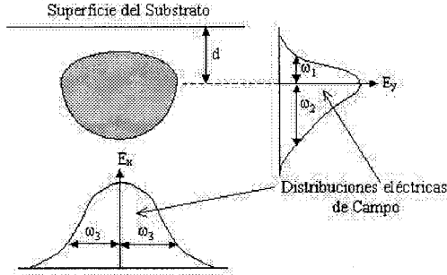
Figura 2: Perfil típico del modo que emerge de la guía de onda.
