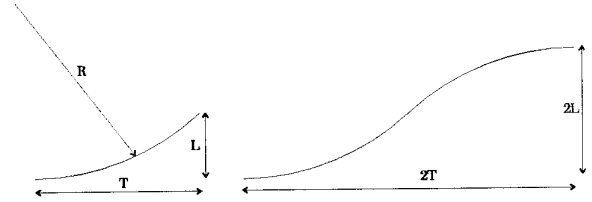
Figura 5: En la figura se exhibe el desplazamiento longitudinal T , el corrimiento lateral L y el radio de curvatura R de un arco de circunferencia, base del diseño de las curvas del derivador propuesto. Los elementos no están a escala.
