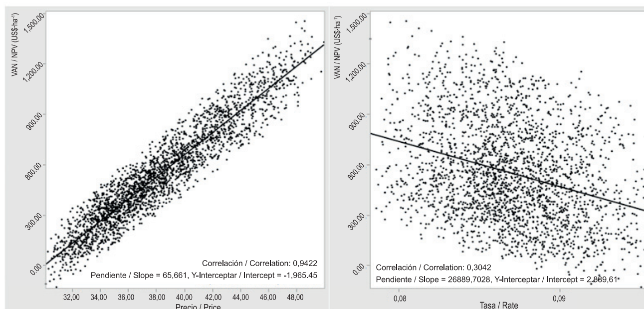
FIGURA 4. Correlación de los supuestos precio y tasa de descuento con el pronóstico para la rentabilidad de la plantación de Eucalyptus globulus con una densidad de plantación de 1,000 árboles- \text{ha}^{-1} .
