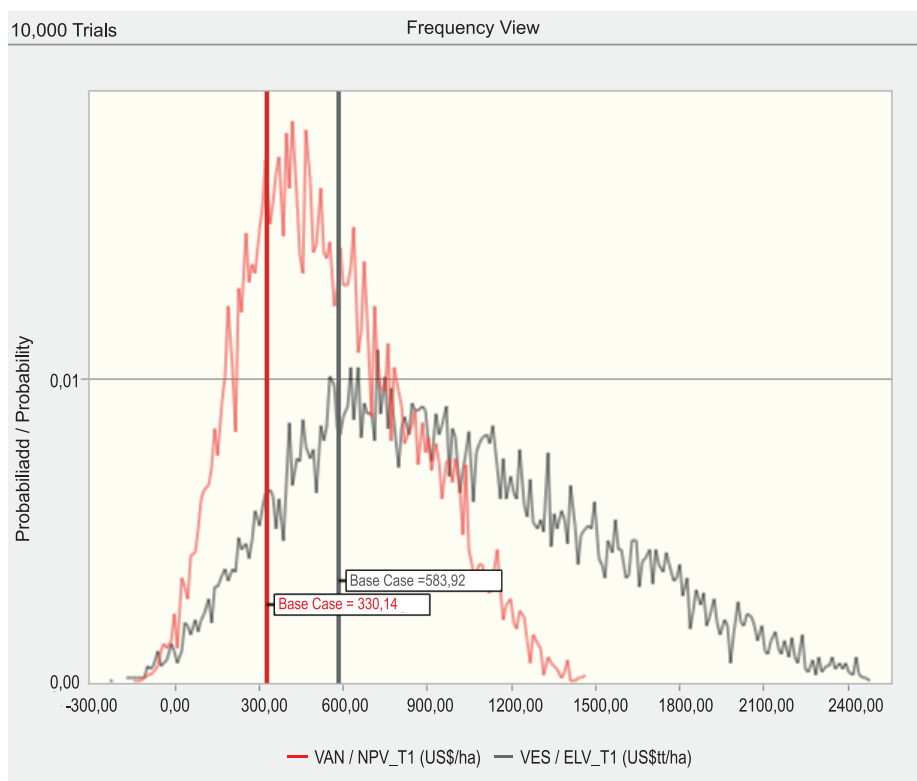
FIGURA 3. Distribución de frecuencias del valor actual neto (VAN) y valor económico del suelo (VES) obtenidos con la simulación de Montecarlo, para una densidad de plantación de 1,000 árboles- \text{ha}^{-1} (T1) de Eucalyptus globulus .
