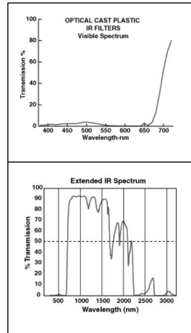
Figura 5. Respuesta de transmisión del filtro
