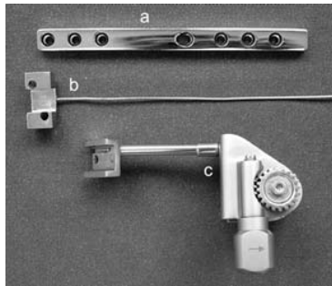
Figura 1 - Os elementos do sistema de transporte: (a) placa, (b) carro móvel, (c) dispositivo tracionador.
