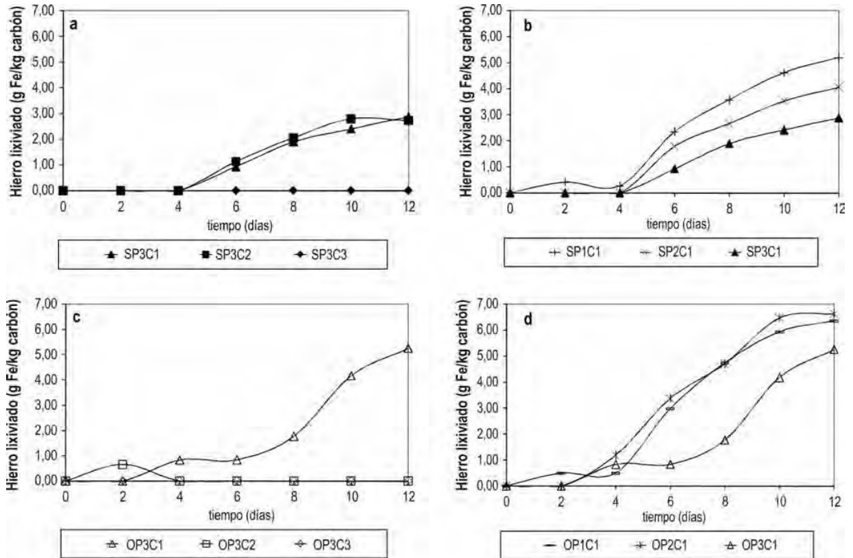
Figura 6. Hierro lixiviado vs. tiempo, ensayos de biodesulfurización de carbón: variación en la concentración de hierro inicial, pH inicial 1.7, tamaño de partícula -malla 60 (a) y -malla 8 (c) y variación en el pH inicial, concentración de hierro inicial 200 ppm, tamaño de partícula -malla 60 (b) y -malla 8 (d).
