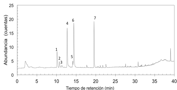
Figura 3: Perfil cromatográfico del aceite esencial de romero. Picos 1 a 7 detallados en Tabla 1.
