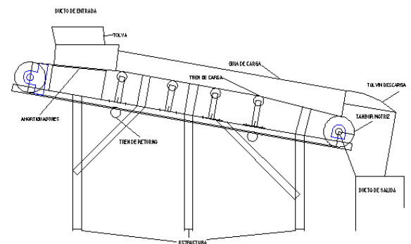
Figura 4. Sistema de banda transportadora
