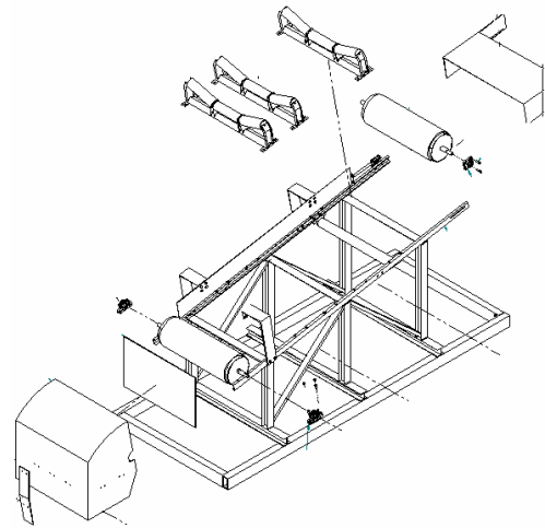
Figura 6. Estructura y tambores de soporte de banda transportadora
