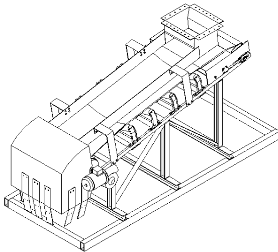
Figura 8. Sistema de transporte por banda, montaje completo
